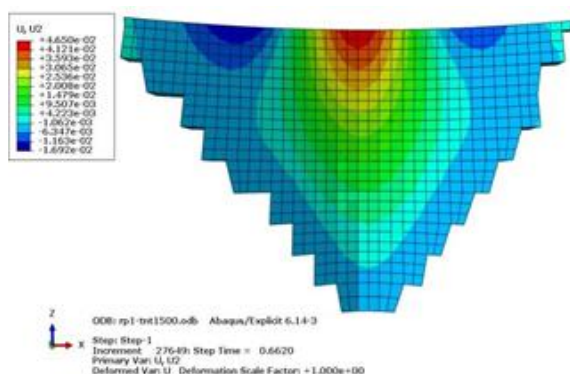
شکل (۱۸): کانتور حداکثر تغییر مکان افقی تاج سد تحت اثر انفجار برای حالت مخزن پر
