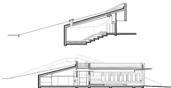
شکل (۲۰): مقطع از مرکز بازدید رامت حنادیو [۴۲]
