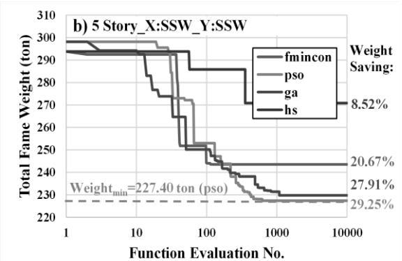
شکل (۶): جزئیات همگرایی چهار الگوریتم بهینه‌سازی.
