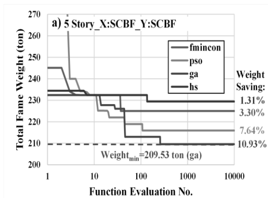
شکل (۴): جزئیات همگرایی چهار الگوریتم بهینه‌سازی.
